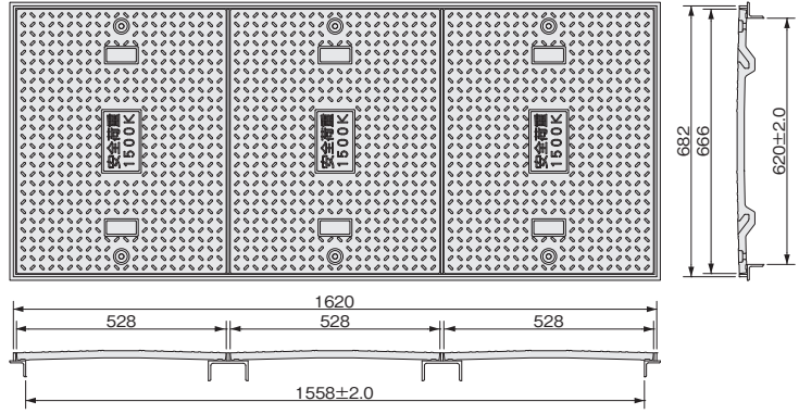
666×528蓋3枚使用 有効開口寸法620×1558
