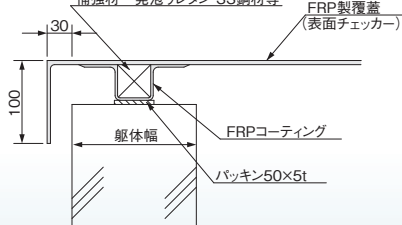
蓋据付断面参考図(開口寸法が大きい場合)
