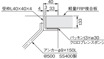
軽量FRP複合板 受枠施工詳細図
