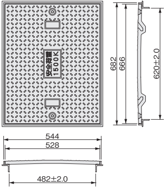
666×528蓋1枚使用 有効開口寸法620×482
