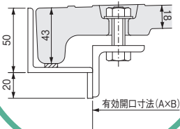
タイプⅡ蓋 受枠断面詳細図
