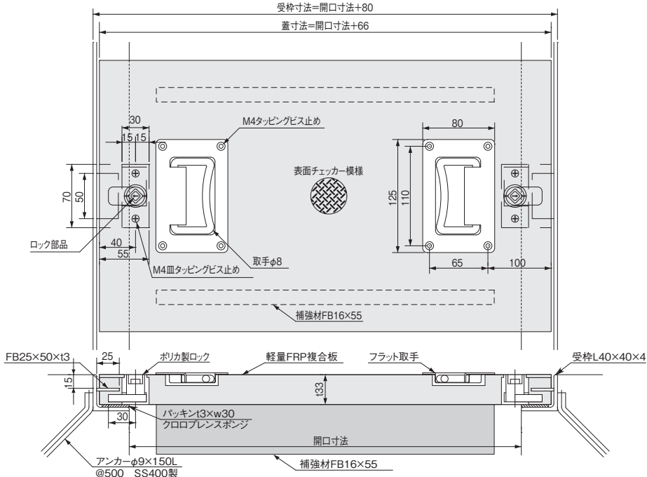
軽量FRP複合板 受枠施工詳細図
