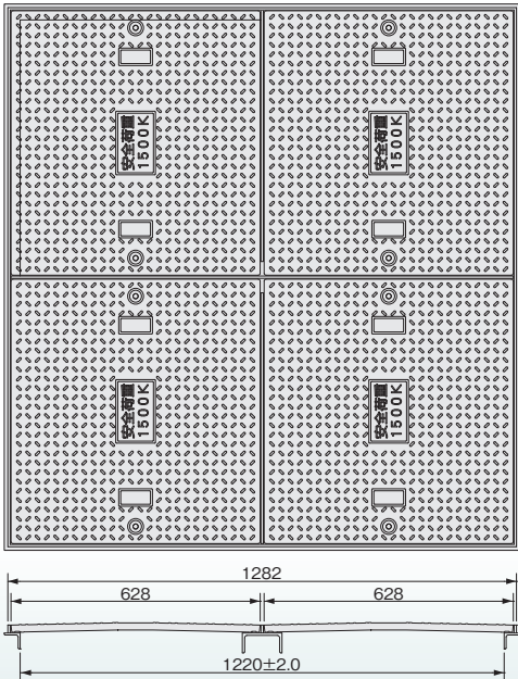
666×628蓋4枚使用 有効開口寸法1296×1220
