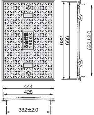
666×428蓋1枚使用 有効開口寸法620×382
