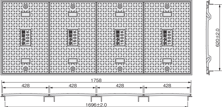
666×428蓋4枚使用 有効開口寸法620×1696
