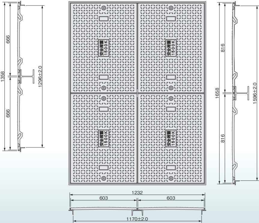
816×603蓋4枚使用 有効開口寸法1596×1170
