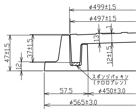
蓋・受枠断面詳細図
