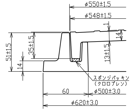
取手断面詳細図
