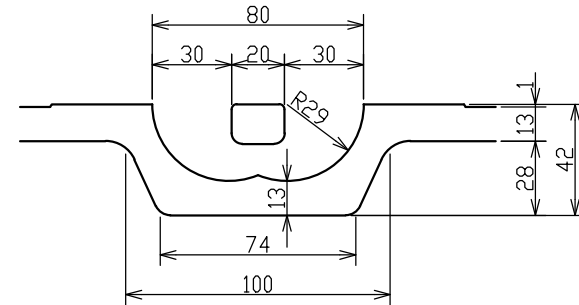
取手断面詳細図
